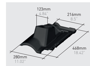
Q132*K | Selectum chimney support klinker
