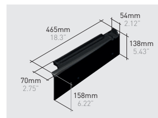
Q134*K | Selectum right side course klinker
